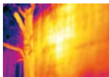
Edifici: presenza d'acqua e muffa
