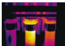
Impianti elettrici: fusibili surriscaldati
